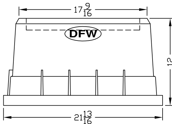
DFW1200TTX.12.BODY
