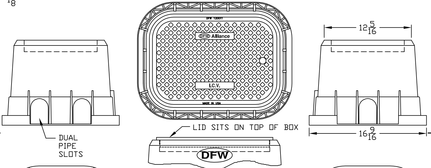
DFW1200TTX.12.1
