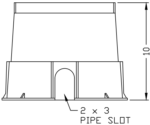
DFW1100.10.BODY
