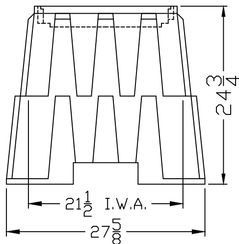
DFW1730FH-24-BODY
